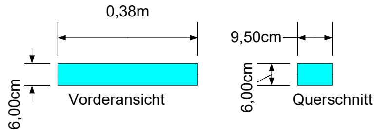
Einzelmodul
