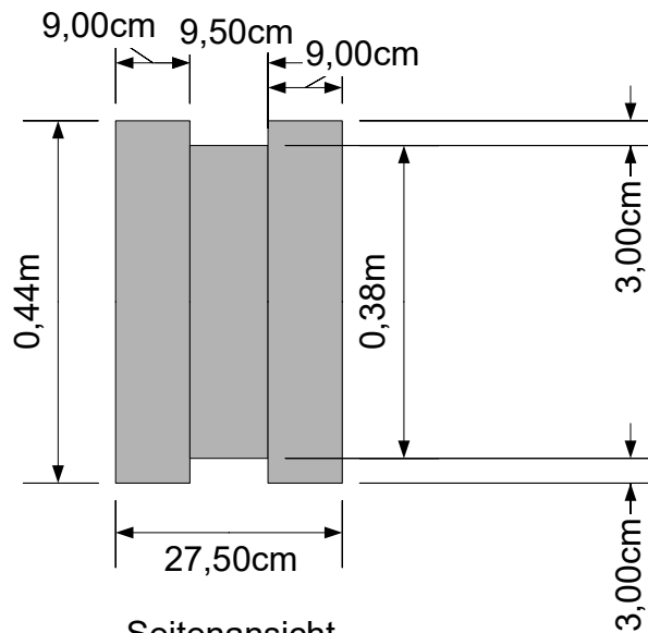
Seitenansicht
